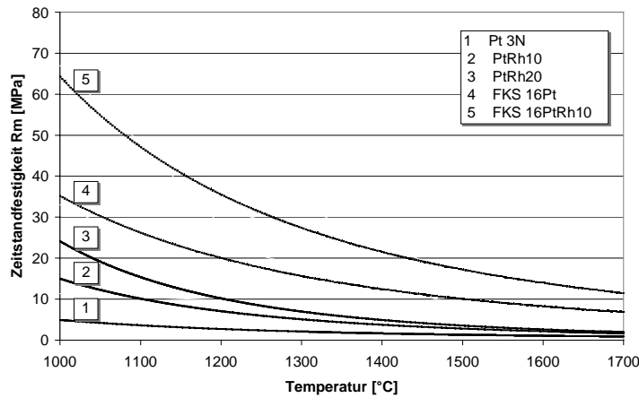
Abbildung 2: Zeitstandsfestigkeit (100 h) verschiedener Platin-Konstruktionswerkstoffe als Funktion der Temperatur
