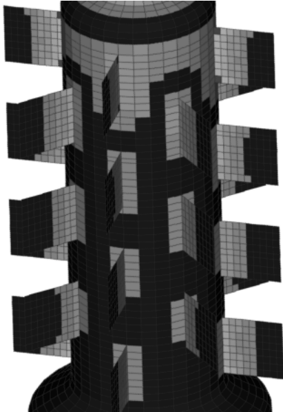
Abbildung 6: Spannungsverteilung Keulenplunger
