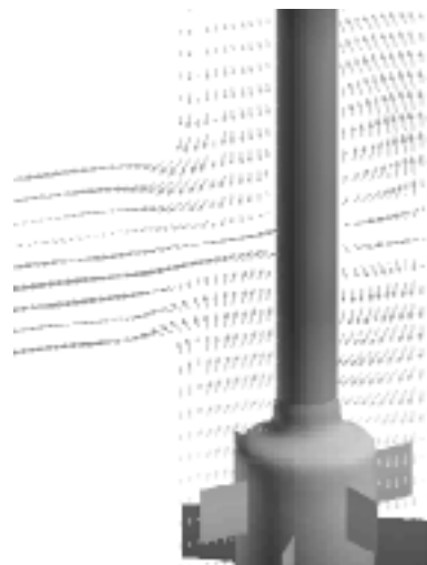
Abbildung 5: Strömungsverhältnisse Feederzelle
